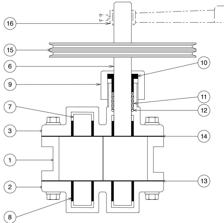
A矢視図(断面図)
