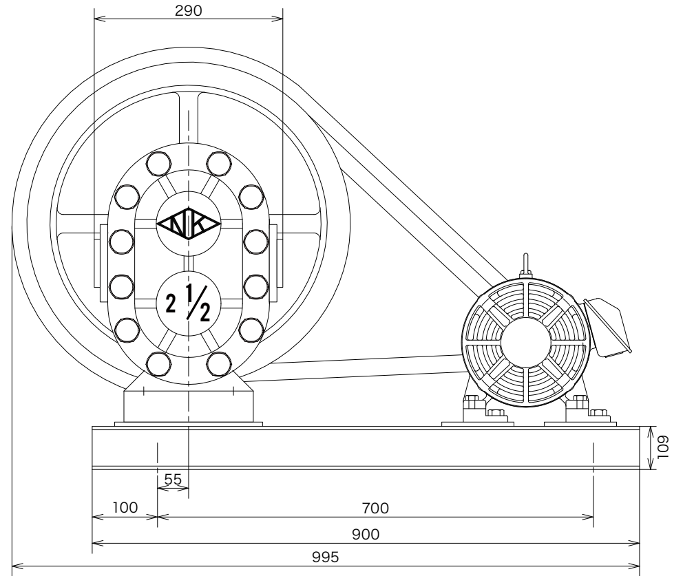
ポンプ側Vプーリ (P.P) 18×A3 / モーター側Vプーリ (M.P) 3 1/2×A3 / VベルトA 77
