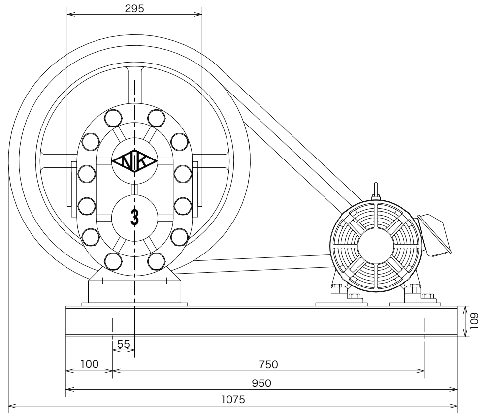
ポンプ側Vプーリ (P.P) 20×B3 / モーター側Vプーリ (M.P) 4×B3 / VベルトB 85
